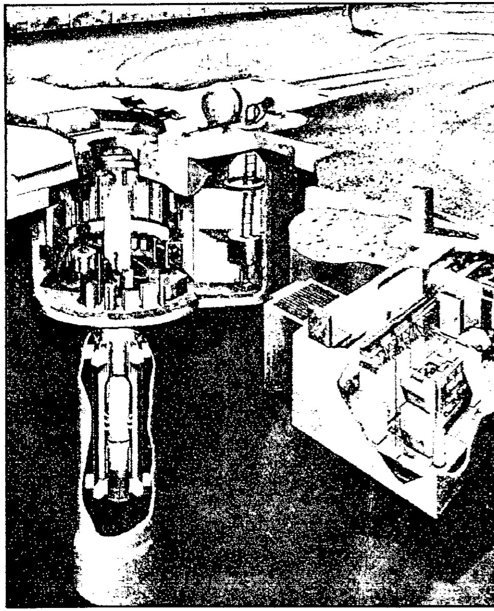
قطع توضيحي لوصلة الصاروخ الاميركي العاب للقطارات «نيوتمان» المائل لصوامع الصواريخ السوفيتية «اس اس - ١٨».
